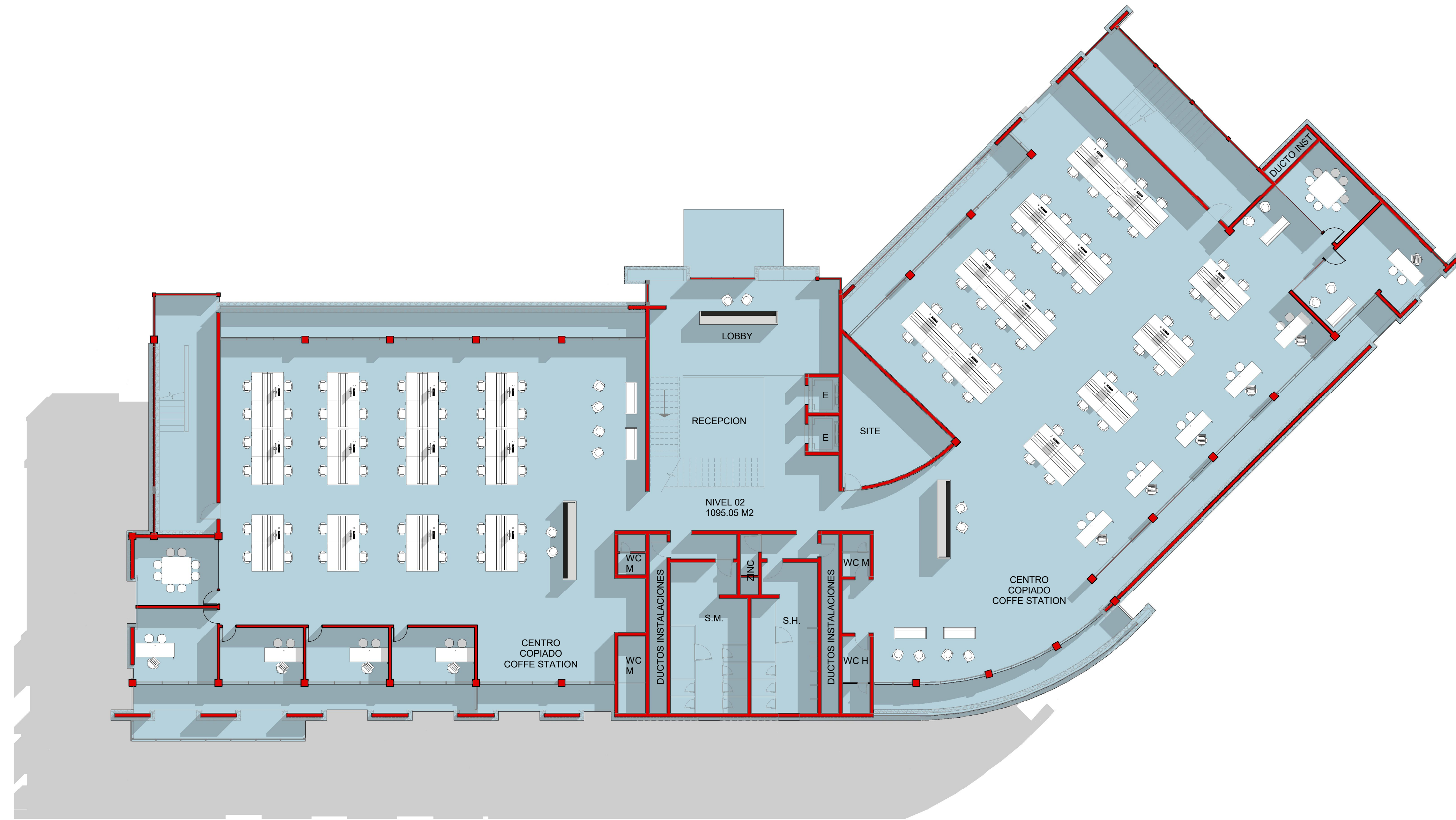
1 Planta Arquitectónica N02 A103 1 : 150
